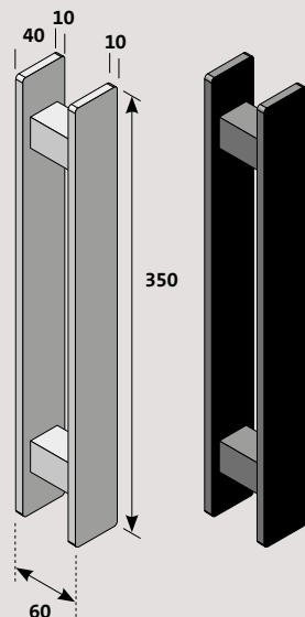
Griffstange Eckig
