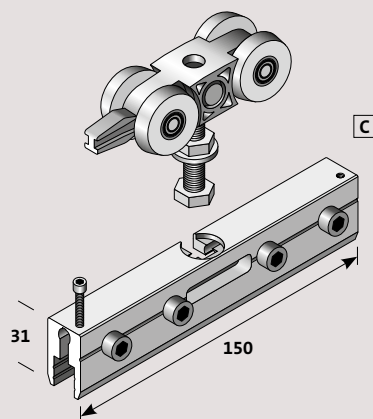
Alu-Klemmbacke mit Türstopper-Laufwagen
