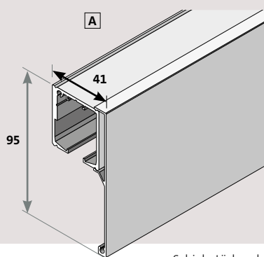
Schiebetürbeschlag
