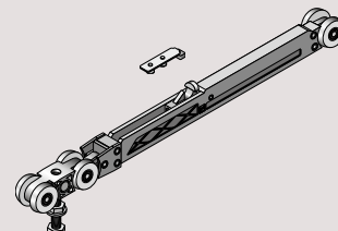
Selbsteinzug-Laufwagen
