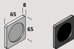
Griffmuschel Quadratisch/Rund
