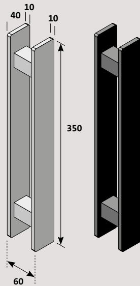
Griffstange Eckig
