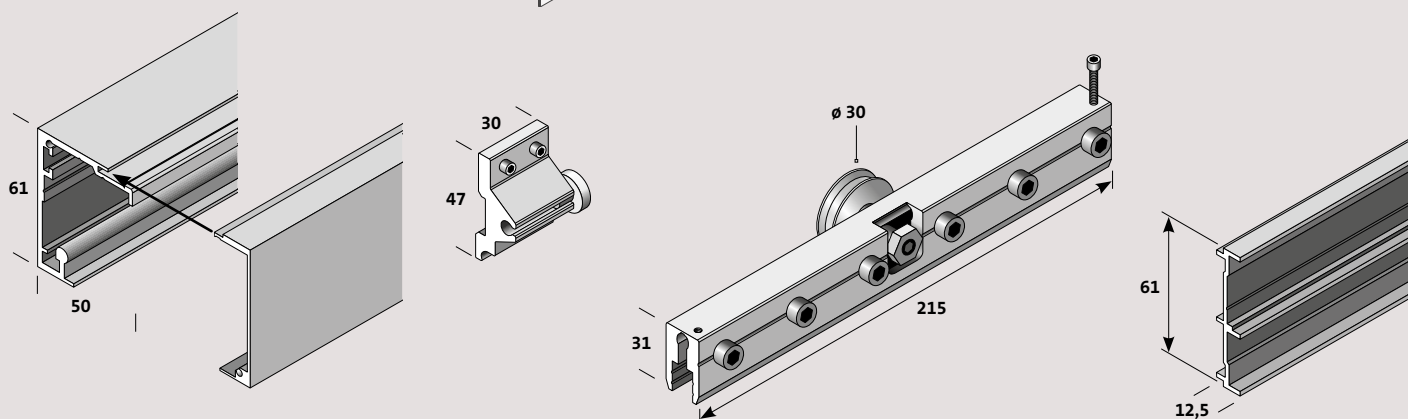
Alu-Laufschiene
