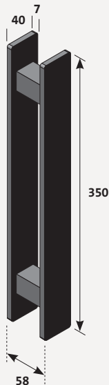
Griffstange Eckig
