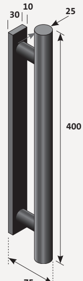
Griffstange Gerundet
