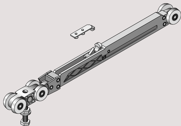
Selbsteinzug-Laufwagen
