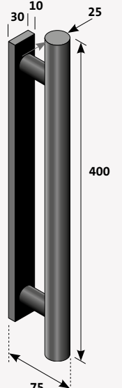
Griffstange Gerundet
