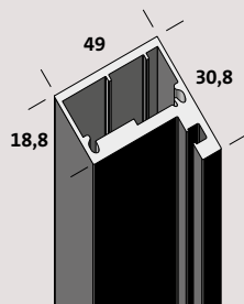
Blockzarge für Drehtür stumpf einschlagend
