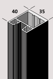
Türrahmen stumpf einschlagend
